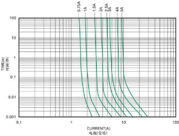
0603FT RoHS I-T CHARACTERISTICS CURVE 0603FT RoHS 电流-时间曲线图
